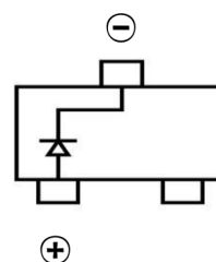
SOT-323
