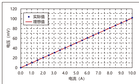
CSFR1206 尺寸 10mΩ 样品
